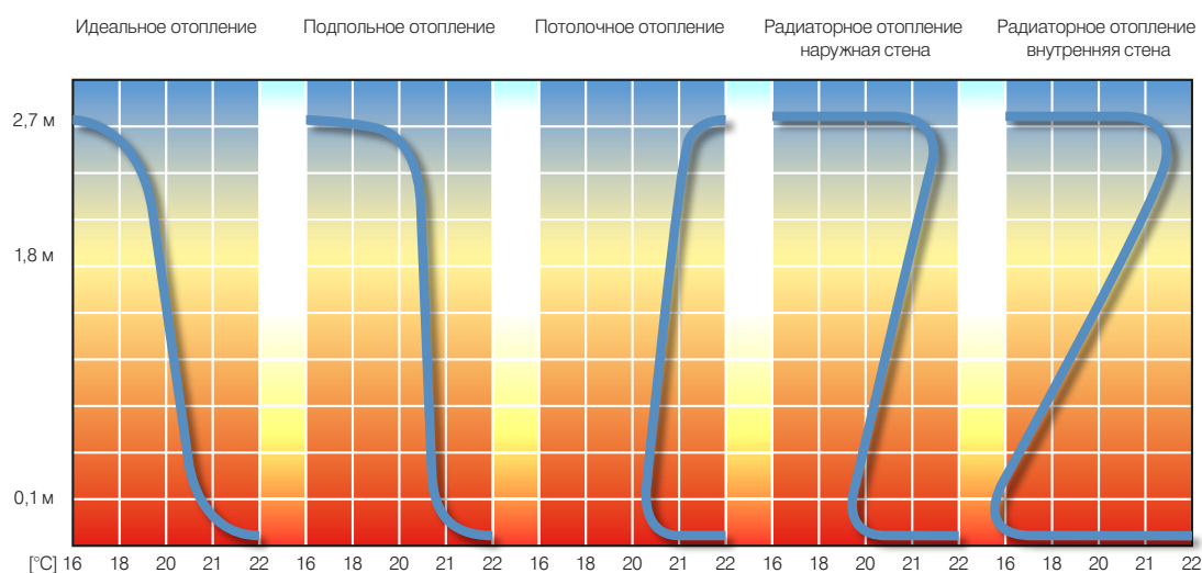
Рис. 1. Вертикальное распределение температуры для разных типов отопления
