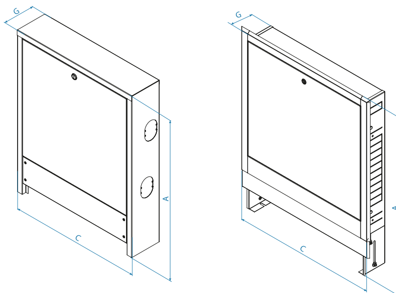
Рис. 52. Размеры монтажных шкафчиков KAN-therm
