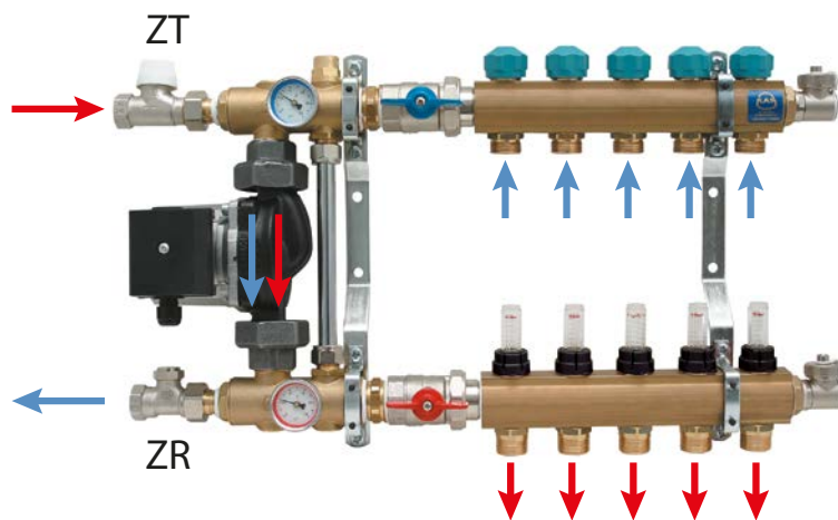
Рис. 60. Распределитель со смесительной системой серии 77A (или 73A) – направления потоков воды
