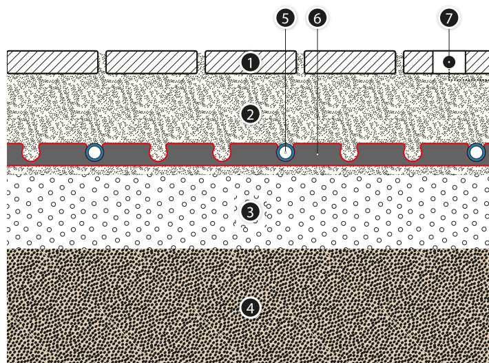
Рис. 39. Подогрев наружных коммуникационных трасс (Система KAN-therm Rail)
