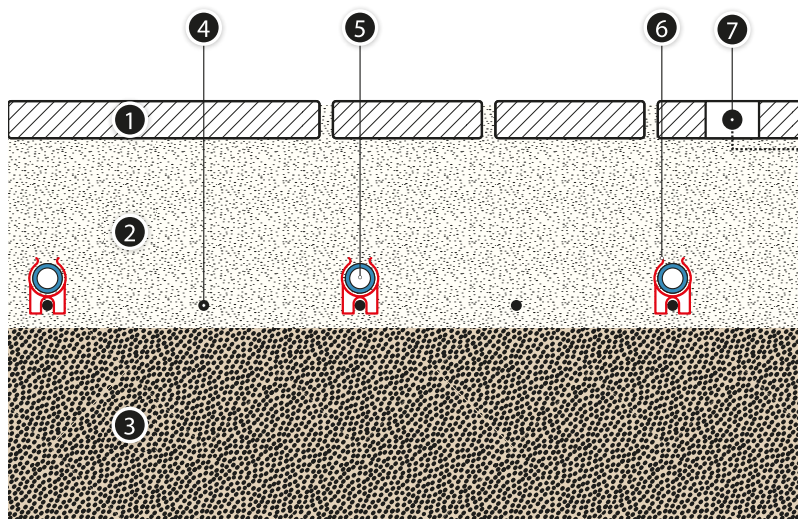
Рис. 40. Подогрев наружных коммуникационных трасс (Система KAN-therm NET)
