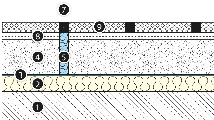
Рис. 15. Выполнение разделительного шва в случае напольного покрытия в виде плитки из камня.
