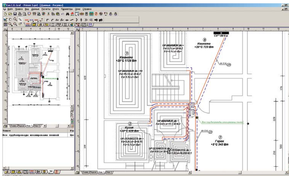
Рис. 81. План этажа с нанесенными подпольными отопительными приборами.
