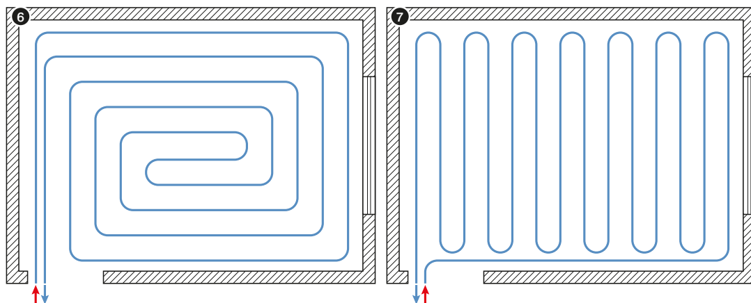
Рис. 6. Контур подпольного отопления/охлаждения в форме спирали (улитки).
