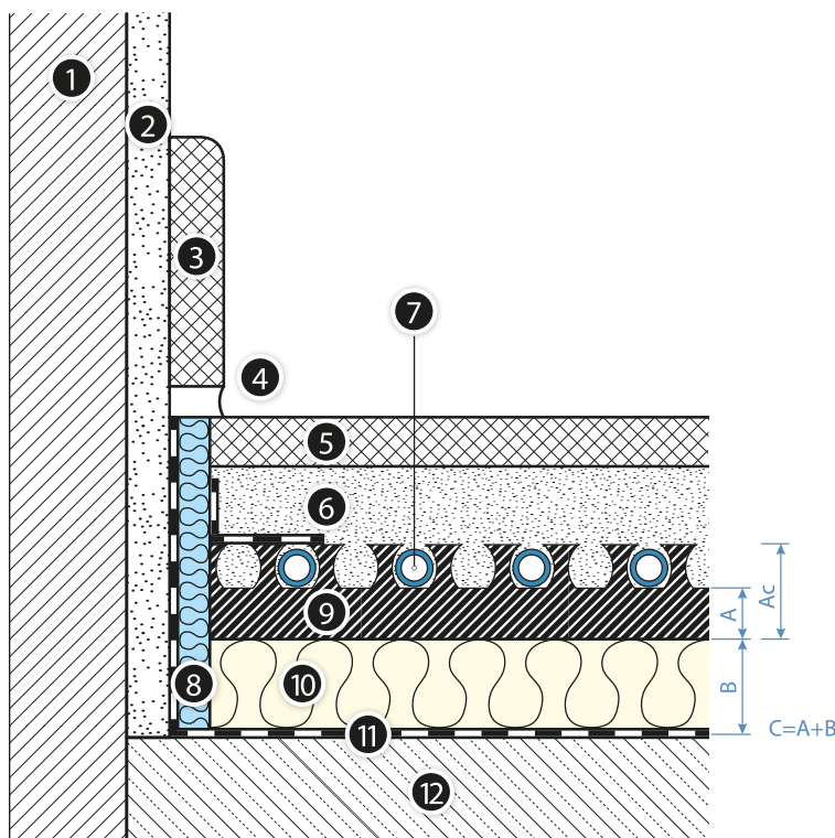
Рис. 28. Подпольный отопительный прибор с системной плитой KAN-therm Profil и дополнительной изоляцией, а также гидроизоляционным покрытием на перекрытии, лежащем на грунте
