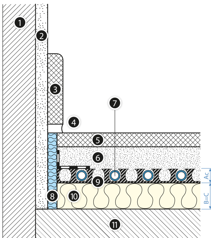
Рис. 27. Подпольный отопительный прибор с системной плитой KAN-therm Profil3 и дополнительной изоляцией на перекрытии над неотапливаемым внутренним помещением, а также на перекрытии, лежащим на грунте (требуется гидроизоляция!)
