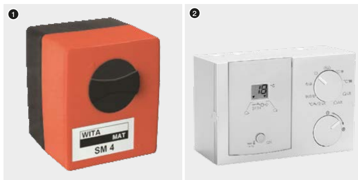
Рис. 56. Управляющие элементы центральной смесительной системы KAN-therm (сервопривод SM4 (1) и погодный регулятор (2))
