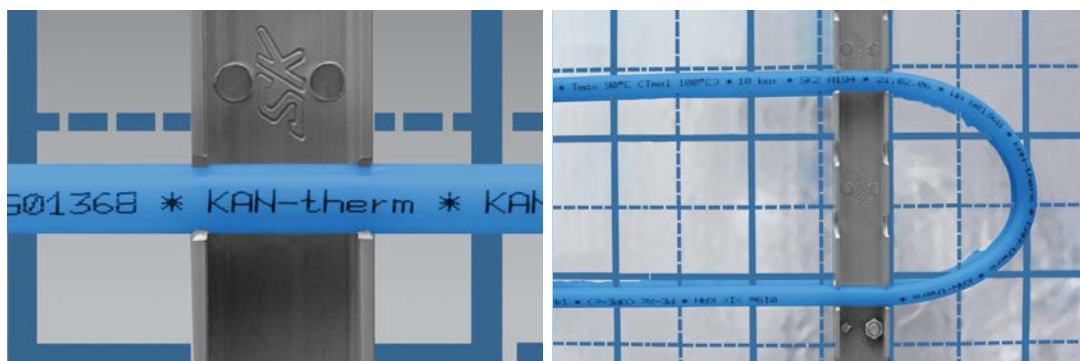
Рис. 33. Крепление греющих труб KAN-therm в стеновом отоплении, выполненным мокрым методом
