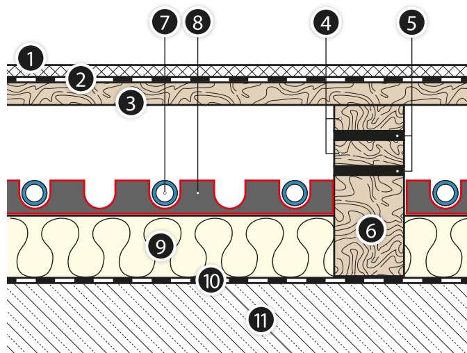
Рис. 38. Конструкция спортивного поверхностно-эластичного пола с системой подпольного отопления, выполненного из элементов системы KAN-therm Rail
