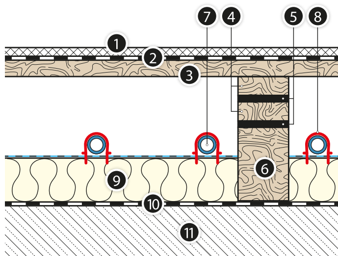
Рис. 37. Конструкция спортивного поверхностно-эластичного пола с системой подпольного отопления, выполненного из элементов системы KAN-therm Tacker.
