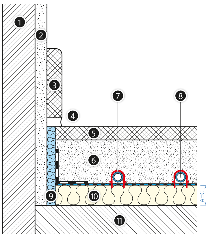
Рис. 21. Подпольный отопительный прибор с системной плитой KAN-therm Tacker на перекрытии над внутренним помещением
