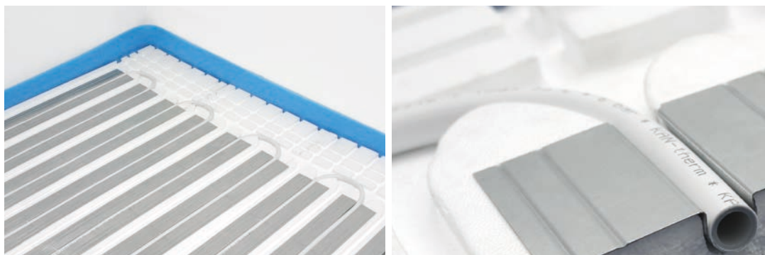
Рис. 36. Плита KAN-therm TBS 14 со стальным излучающим профилем
